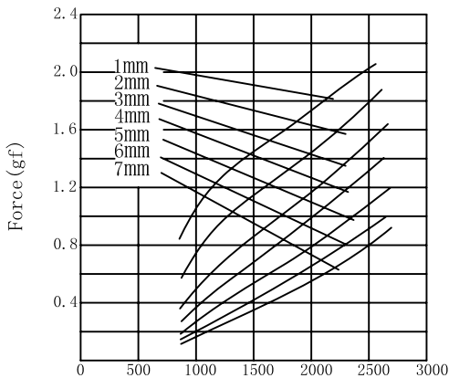
AMPERE-TURNS Vs FORCE 安匝/吸引力
